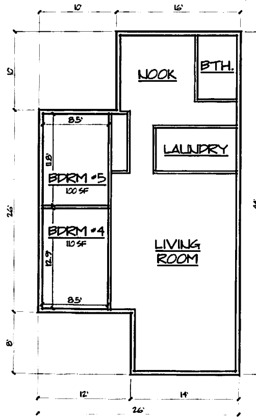
MAIN LEVEL SCALE: 1/8" = 1'-0"
