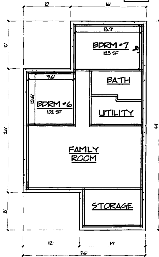
LOWER LEVEL SCALE: 1/8" = 1'-0"
