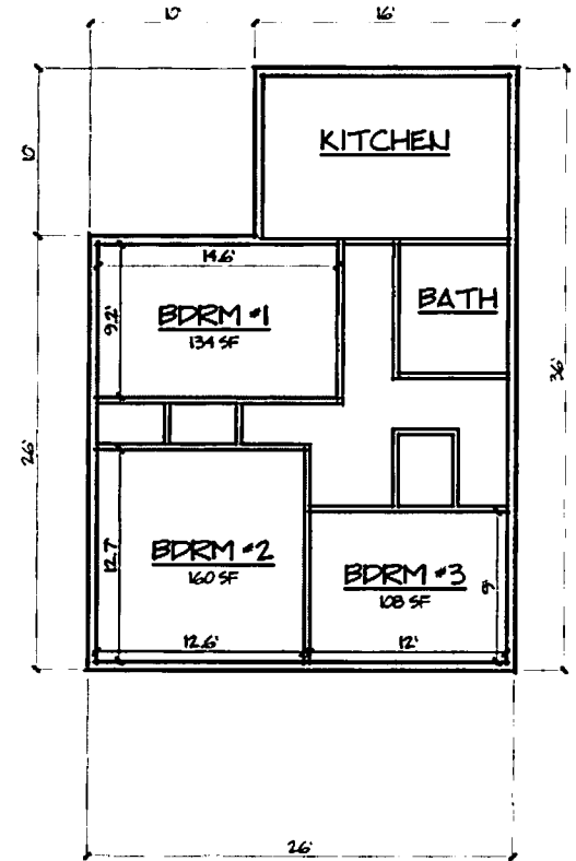
UPPER LEVEL SCALE: 1/8" = 1'-0"
