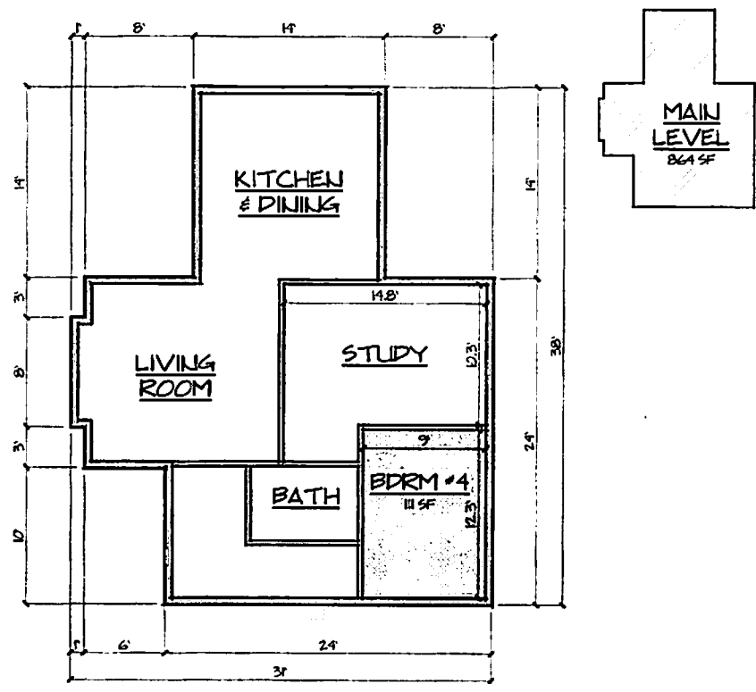
MAIN LEVEL SCALE: 1/8" = 1'-0"
