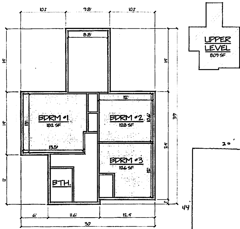
UPPER LEVEL SCALE: 1/8" = 1'-0"
